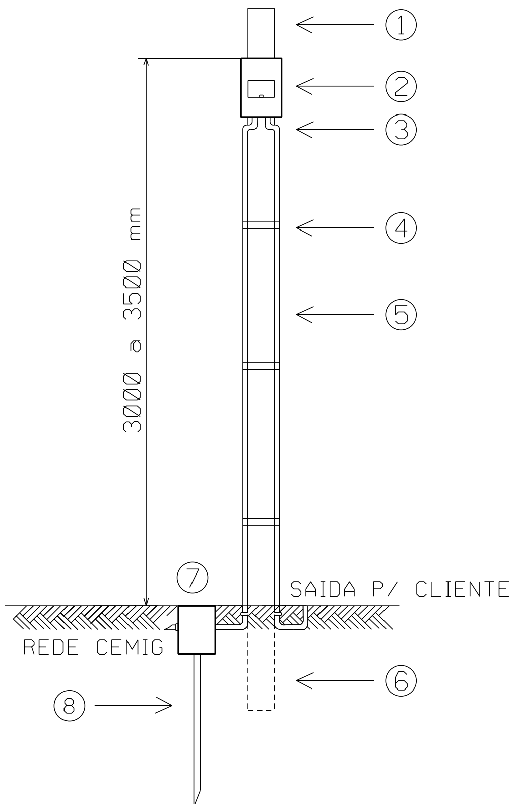
DESENHO 31 - PADRÃO DE ENTRADA COM FORNECIMENTO DE ENERGIA SEM MEDIÇÃO – FSM CASO 5 - REDE DE DISTRIBUIÇÃO SUBTERRÂNEA
