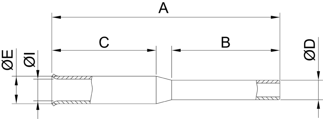
DESENHO 62 - TERMINAL DE COMPRESSÃO VAZADO TIPO PINO
