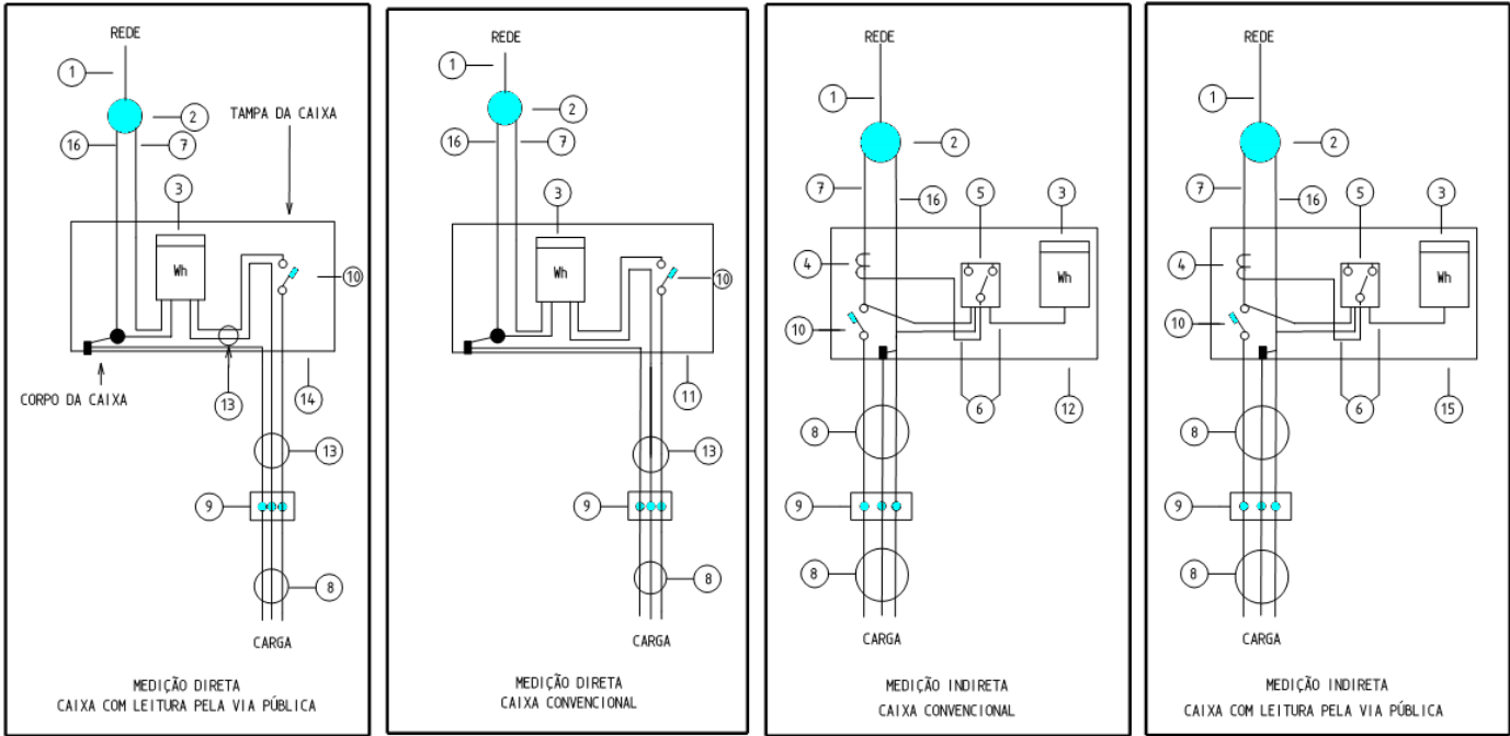
DESENHO 68 - ESQUEMAS DE LIGAÇÃO DOS MEDIDORES DE ENERGIA ELÉTRICA
