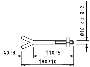
PARAFUSO - CHUMBADOR
