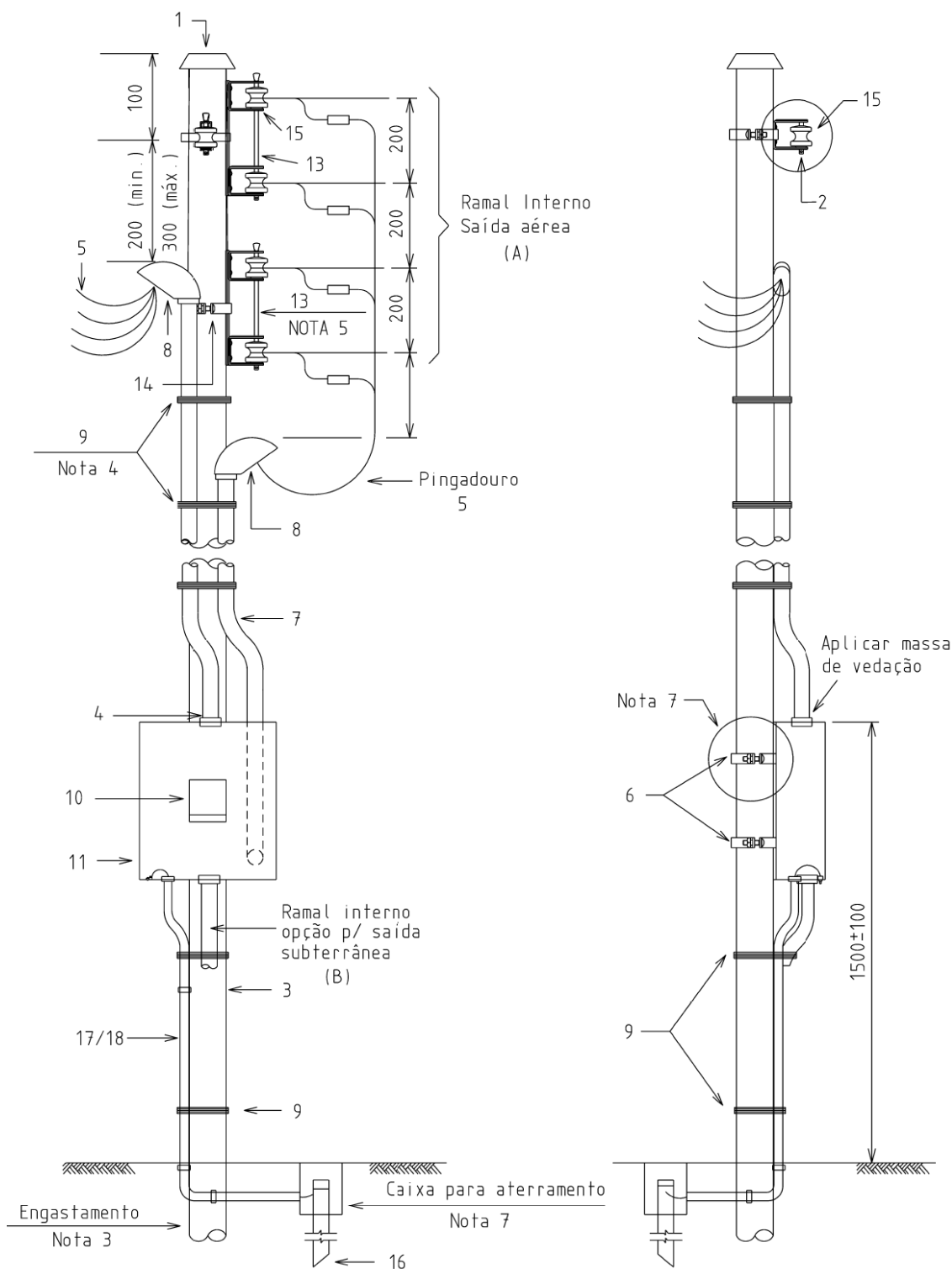
DESENHO 14 - PADRÃO COM RAMAL DE CONEXÃO AÉREO - LIGAÇÃO A 2, 3 e 4 FIOS - CONEXÃO TEMPORÁRIA ATÉ 86 kVA (1 DISJUNTOR DE 225A) – SEM MEDIÇÃO
